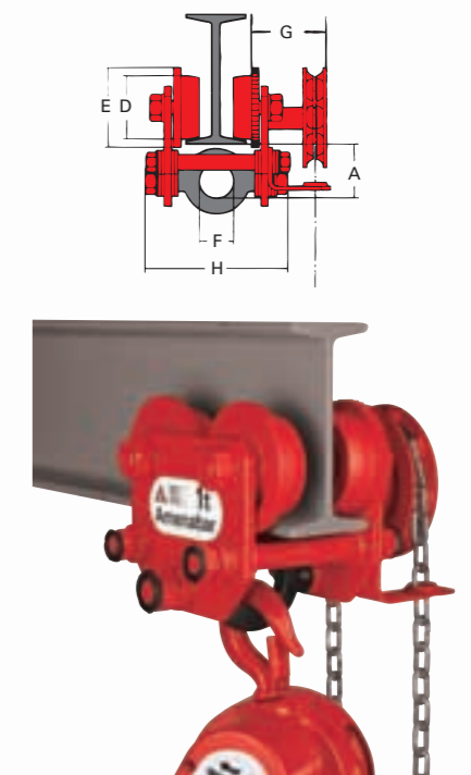
500 to 16.000 Kg. C-T trolley
